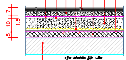
کفسازی بام DET.A
